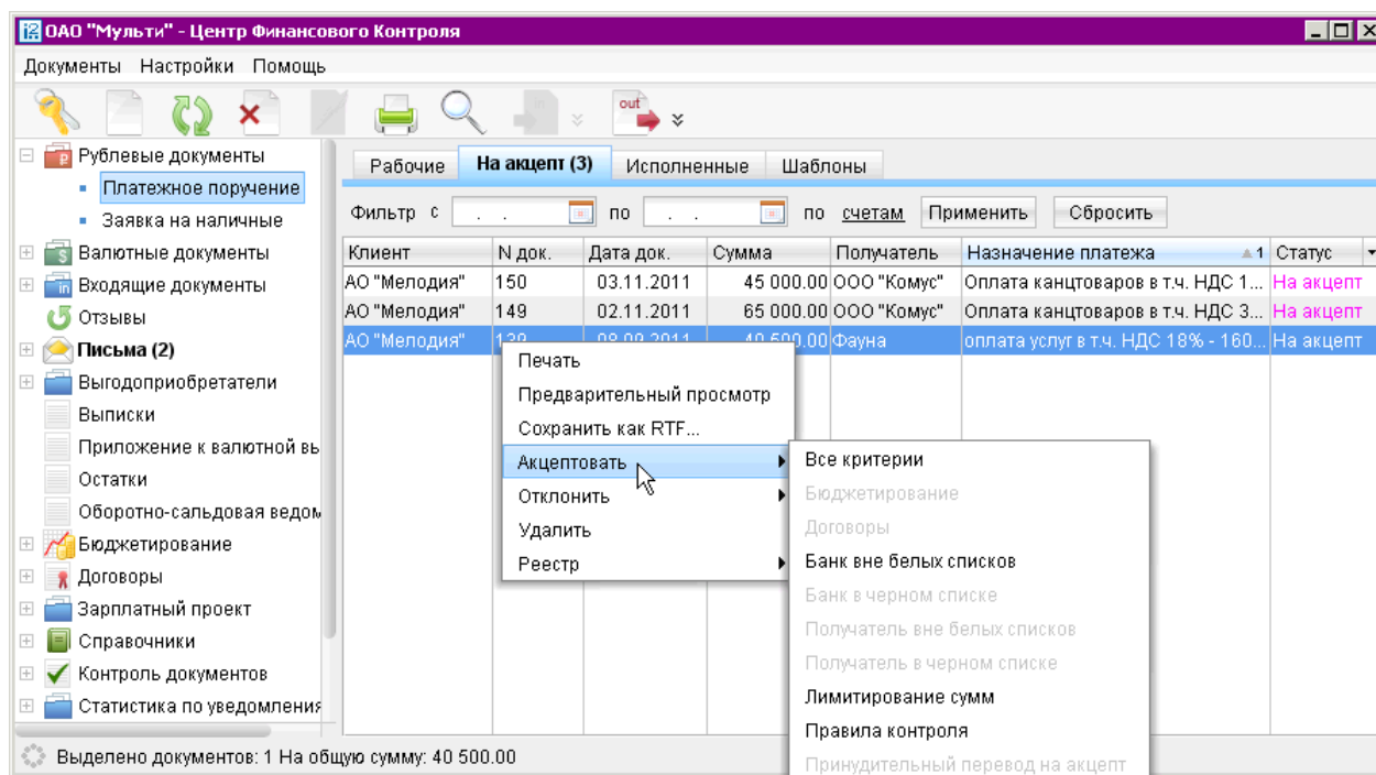
Рис. 11. Акцепт платежей
