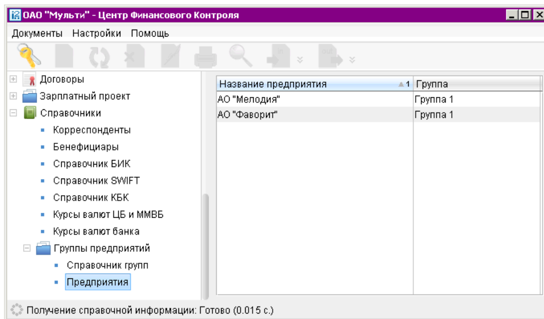
Рис. 33. Ветка Справочники
