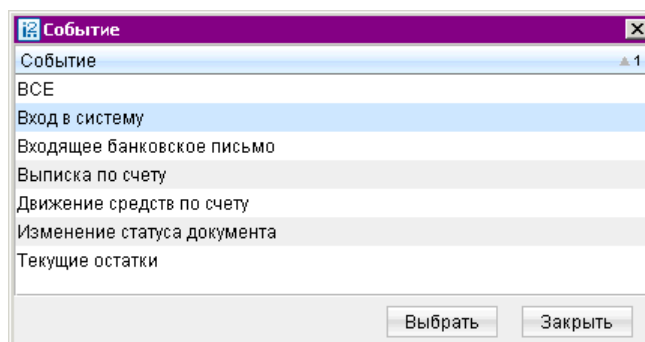
Рис. 43. Окно Событие
