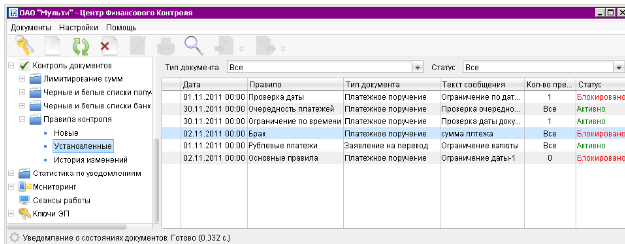
Рис. 31. Раздел Установленные
