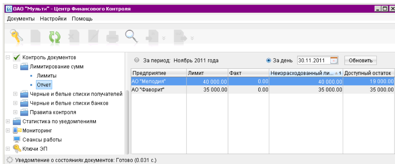
Рис. 17. Раздел Отчет .
